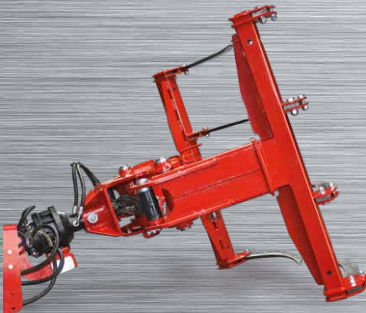
Rotator mit Greiferhochstellung
